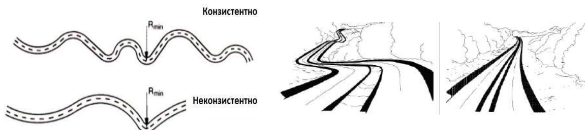
Слика 11.8 – Неконзистентни елементи пружања пута (PIARC, 2009)
