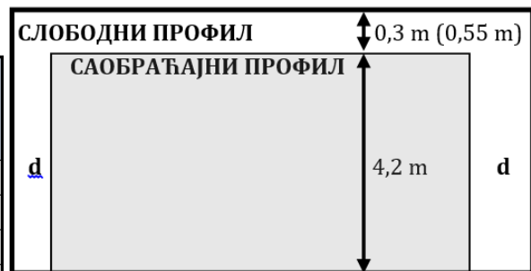
Слика 14.6а – Саобраћајни и слободни профил
