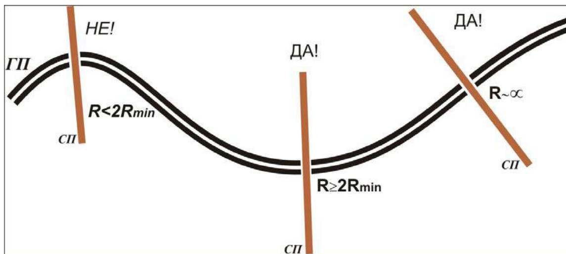
Слика 3.19 – Карактеристични примери могућих позиција укрштаја (прикључка) у односу на ситуациони ток главног правца – извод из Правилника
