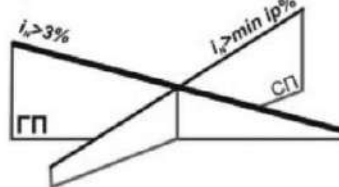
Слика 14.40 – Примери доброг и лошег пружања трасе у зависности од локација укрштања
