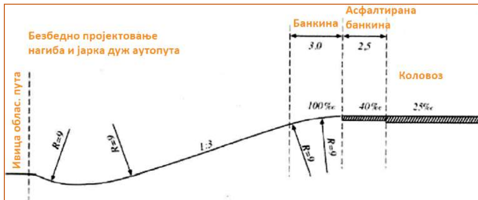
Слика 12.3 – Пројектовање нагиба (ЈП „Путеви Србије“, 2009)
