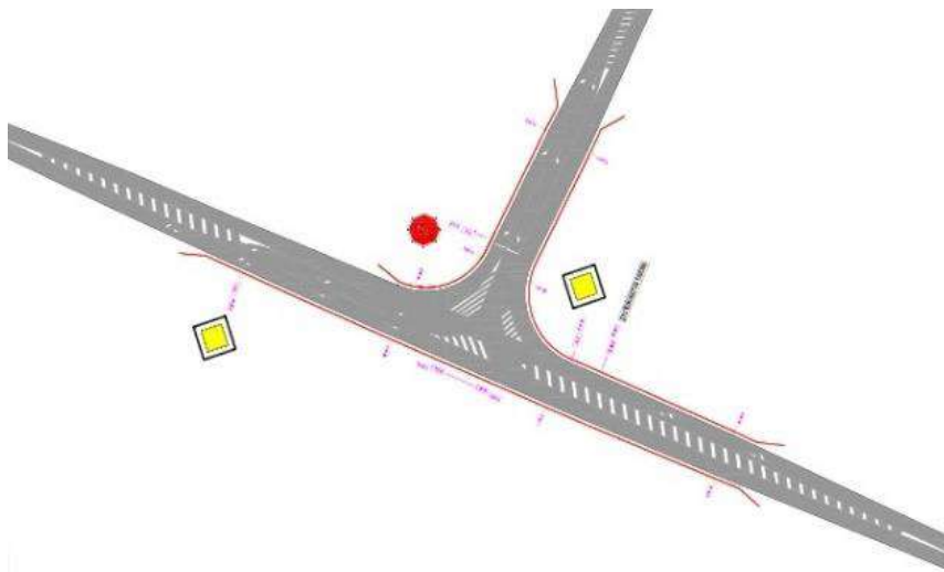
Слика 11.15 – Предложено идејно решење небезбедне „Y“ раскрснице
