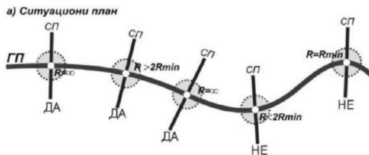
Слика 14.29 – Радијуси траса на местима укрштања
