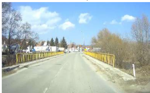
Слика 12.32 – Неадекватна ограда на мосту, недостатак заштитне ограде за возила
