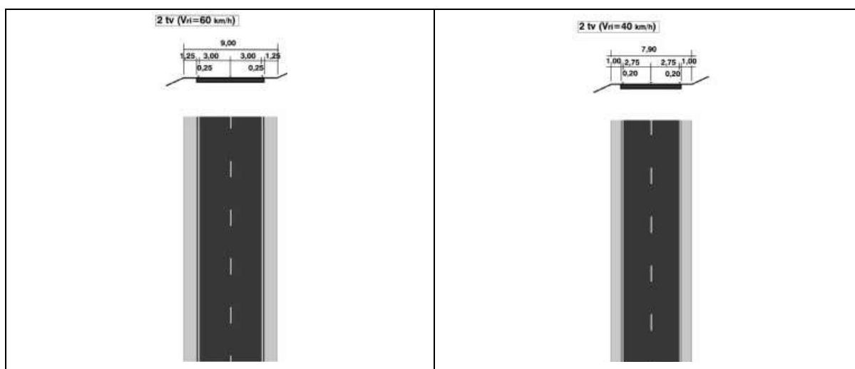
Стандардни ГПП двотрачних путева - П-3 ( V_n=60 \text{ km/h} )
