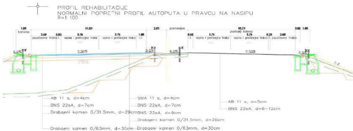
Слика 15.3 – Нормални попречни профил аутопута у правцу на насипу са смањеном ширином коловоза на 10,7 м
