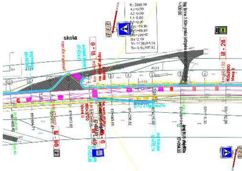
Слика 14.88 – Небезбедан пешачки прелаз у зони школе - овакво пројектно решење не пружа потребну безбедност пешака због непостојања разделног острва, неодговарајућег осветљења као и неадекватног облика „шикана“ дефинисаних пешачких ограда у зони пешачког прелаза
