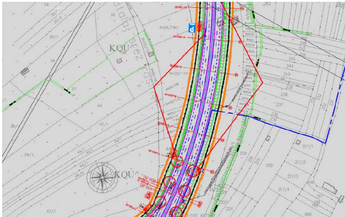
Слика 15.26 – Већи део уливно - изливних трака није обухваћен расветом
