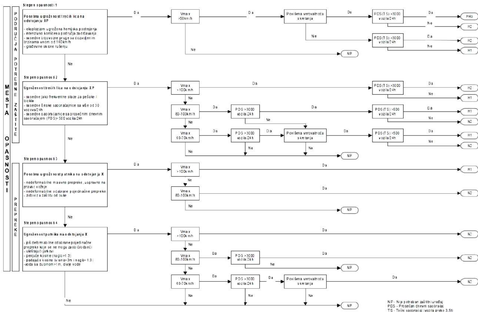
Слика 14.102 – Блок дијаграм за избор степена задржавања заштитног уређаја (Извор: Техничко упутство "Примена система за задржавање возила на државним путевима Р. Србије" - са обавезном применом, ЈП "Путеви Србије", 2011)
