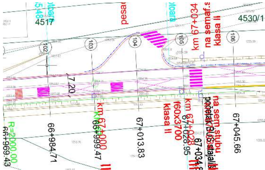
Слика 15.19 – Ближи приказ небезбедног пешачког прелаза
