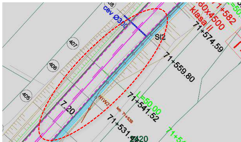
Слика 14.89 – Нефункционалан тротоар - на средини тротоара је предвиђена заштитна ограда услед које се губи функција тротоара
