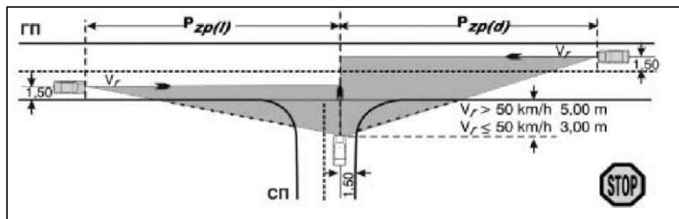
Слика 3.7 – Креирање зоне прегледности на трокракој површинској раскрсници –из Правилника 1
