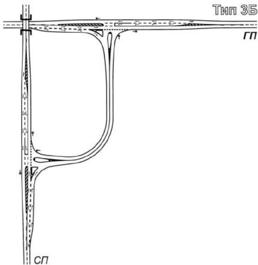
Слика 3.6 – Графички приказ површинских раскрсница ТИП 3Б
