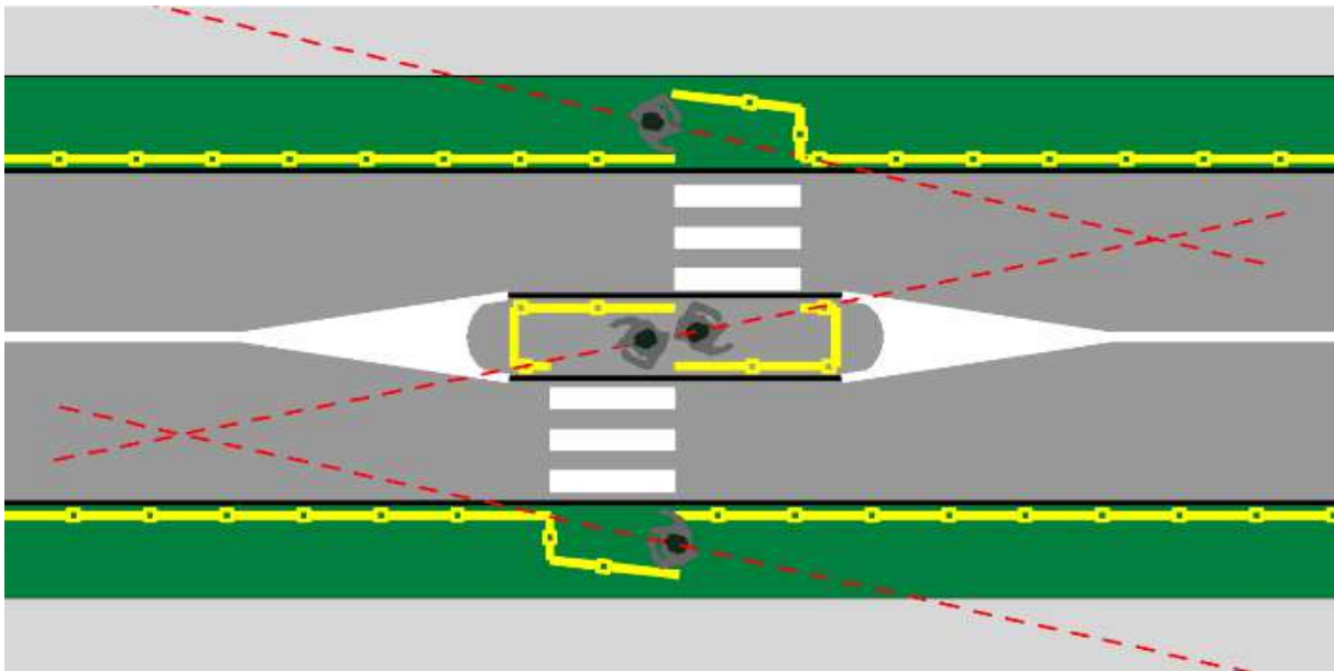
Слика 15.19 - Предлог решења за острво и „шикане“ (скица)
