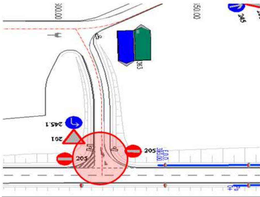
Слика 14.71 – Небезбедно пројектован излаз са станице за снабдевање горивом – кратка трака за искључивање
