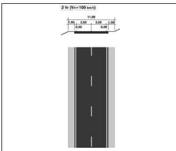
Стандардни ГПП двотрачних путева - П-1 ( V_n=100 km/h)
