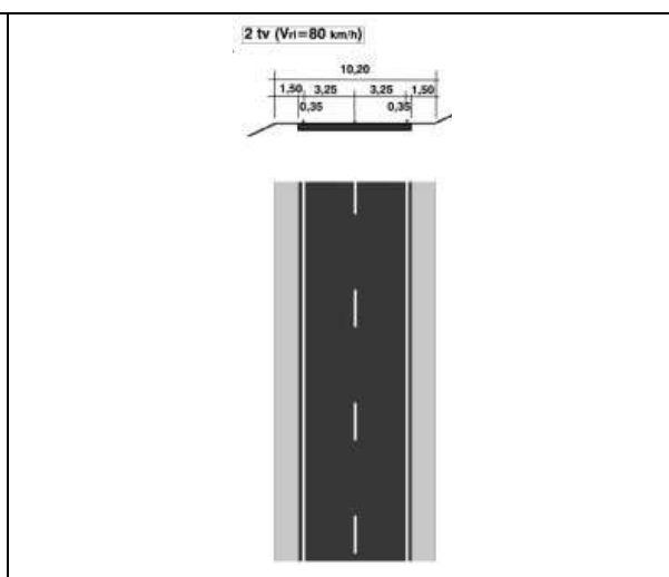
Стандардни ГПП двотрачних путева - П-2 ( V_n=80 km/h)
